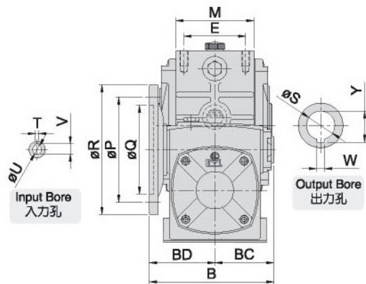
尺寸表 Dimension(m/m)
